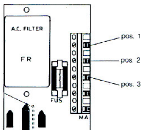
Figura 2-5. Scheda filtro
